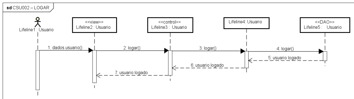
Figura 33 – Diagrama de Sequência – Logar
