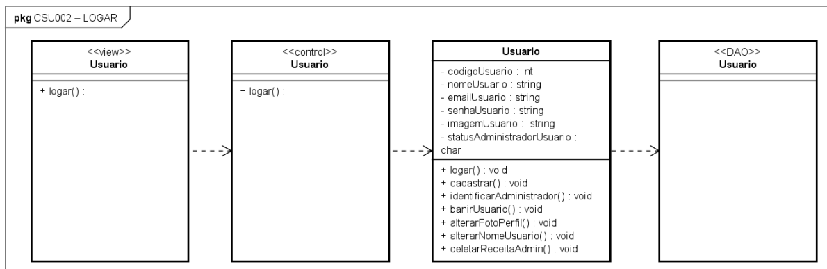
Figura 25 – Diagrama de Classes de Projeto – Logar
