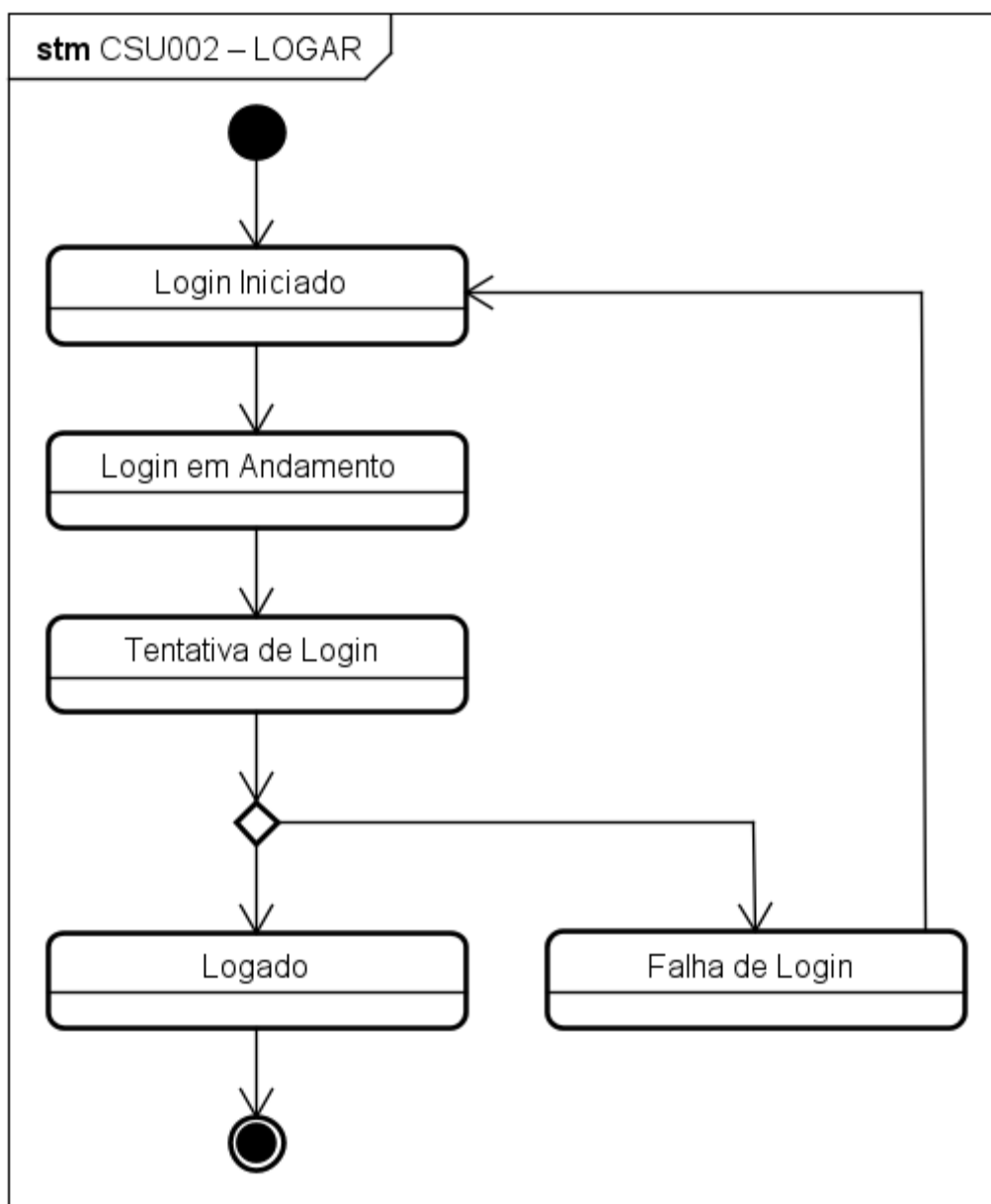
Figura 51 – Diagrama de Estado – Logar
