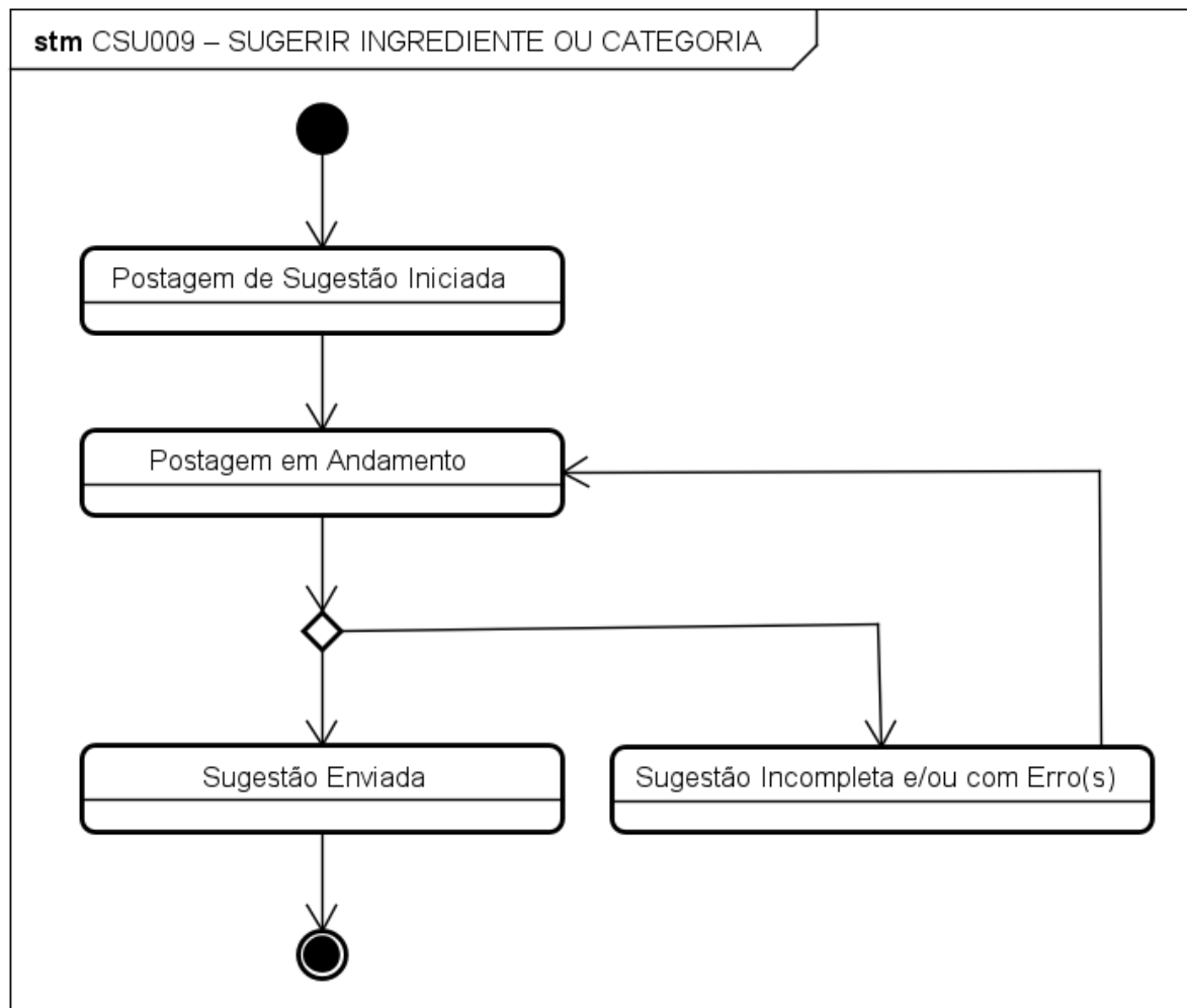
Figura 56 – Diagrama de Estado – Sugerir Ingrediente ou Categoria
