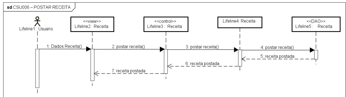
Figura 35 – Diagrama de Sequência – Postar Receita
