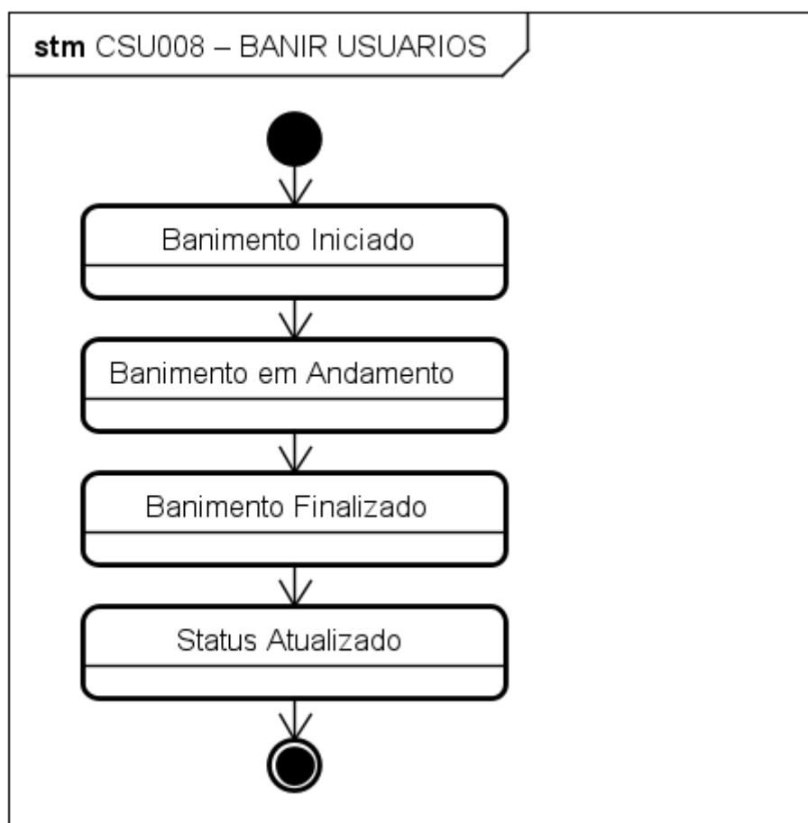
Figura 55 – Diagrama de Estado – Banir Usuário
