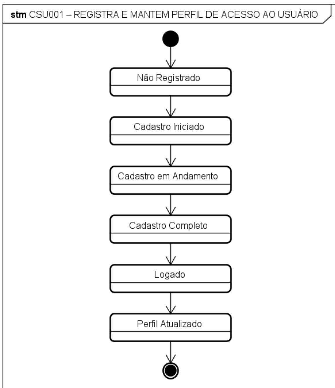
Figura 50 – Diagrama de Estado – Registra e Mantem Perfil de Acesso ao Usuário
