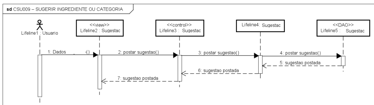
Figura 38 – Diagrama de Sequência – Sugerir Ingrediente ou Categoria
