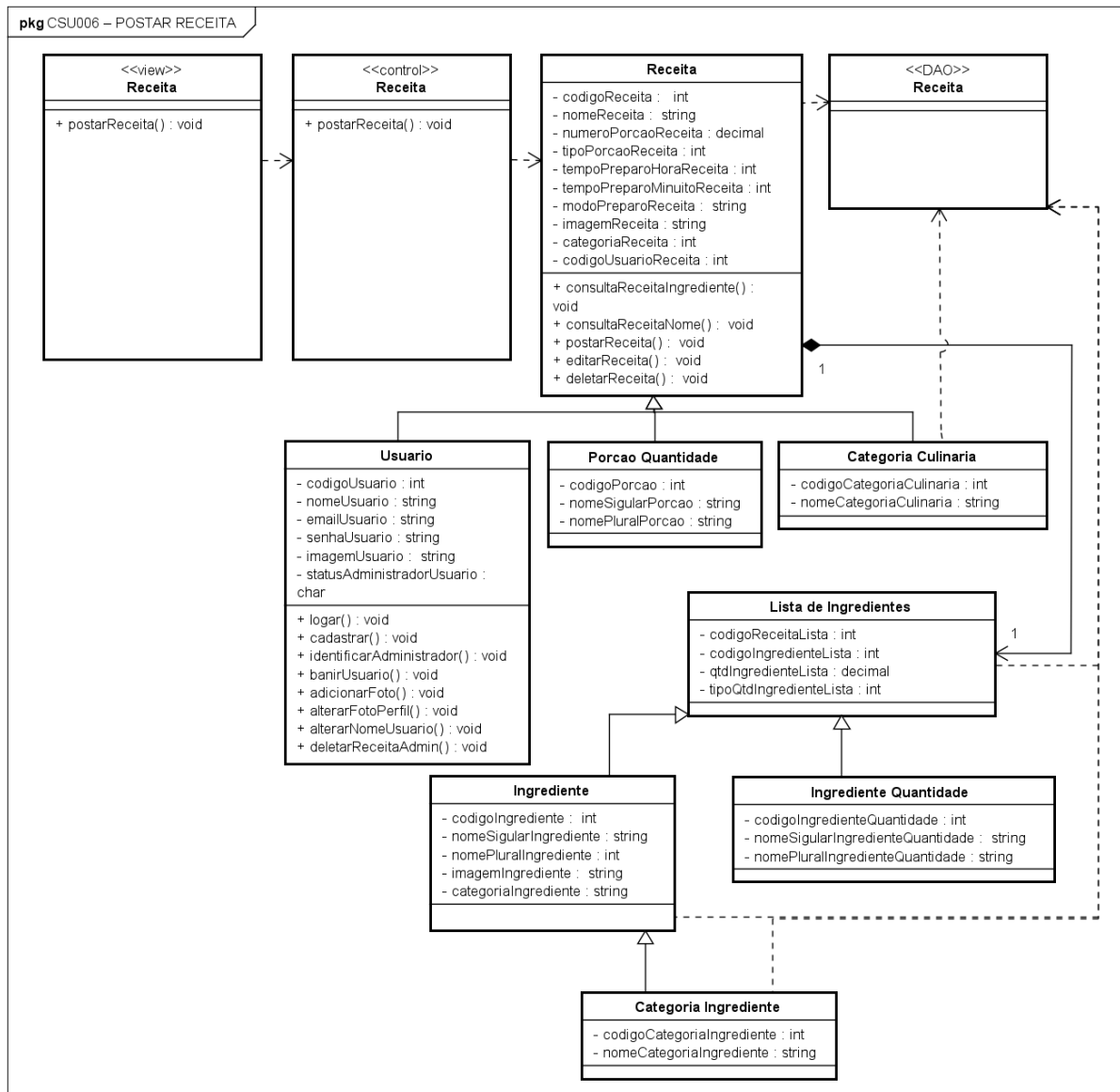
Figura 27 – Diagrama de Classes de Projeto – Postar Receita
