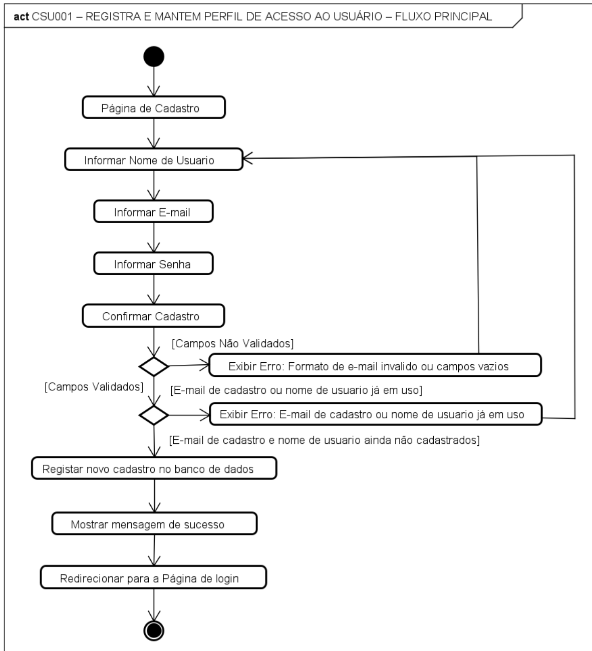
Figura 40 – Diagrama de Atividade – Fluxo Principal do Registra e Mantem Perfil de Acesso ao Usuário
