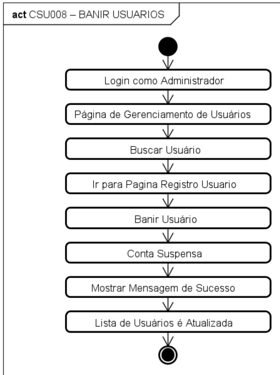
Figura 46 – Diagrama de Atividade – Banir Usuário
