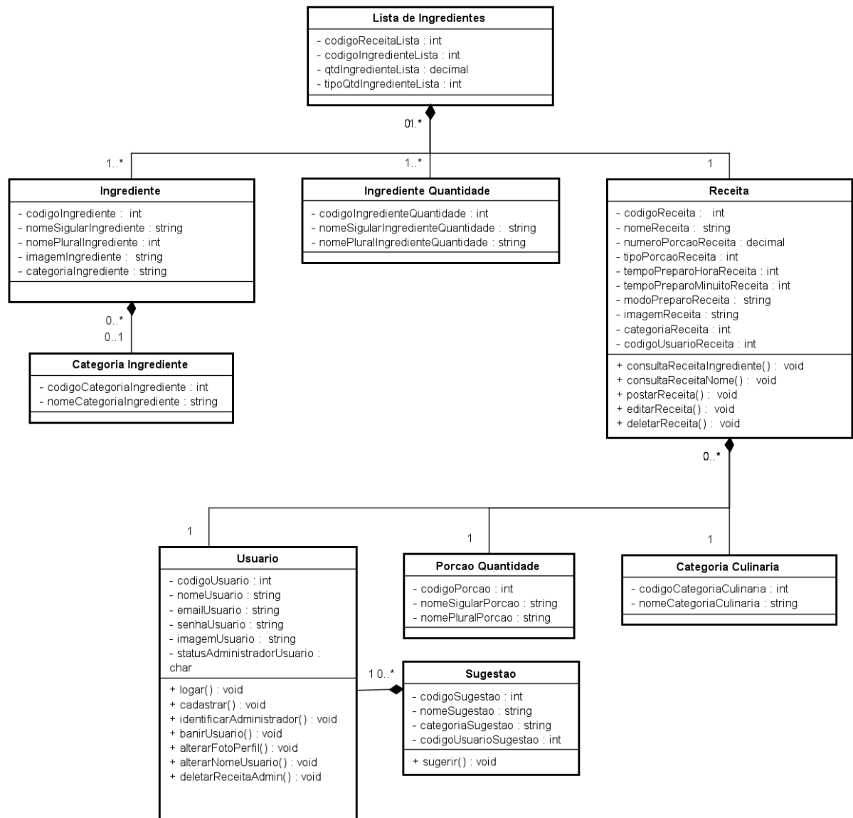
Figura 22 – Diagrama de Classes de Análise (Visão de Negócio)
