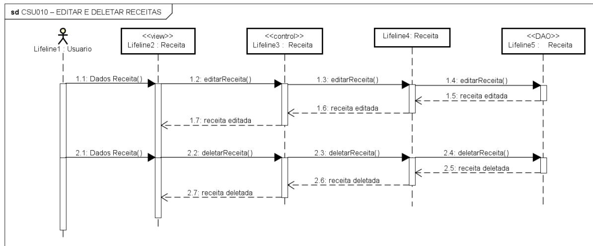
Figura 39 – Diagrama de Sequência – Editar e Deletar Receitas
