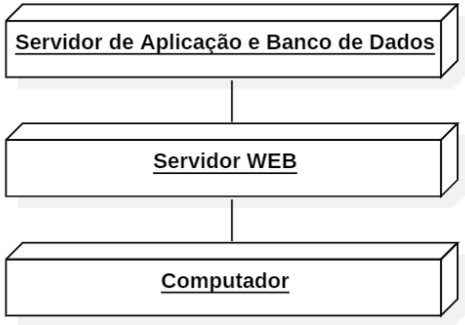
Figura 23 – Diagrama de Implantação
