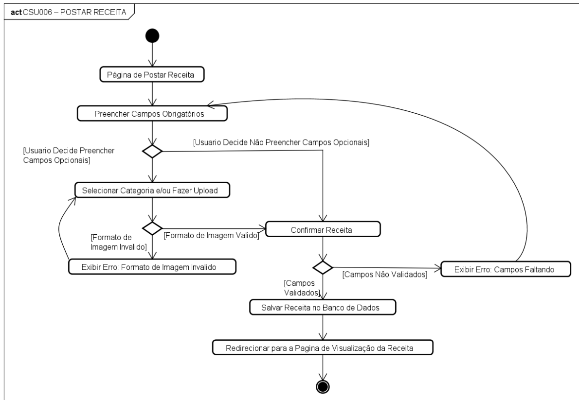
Figura 44 – Diagrama de Atividade – Postar Receita
