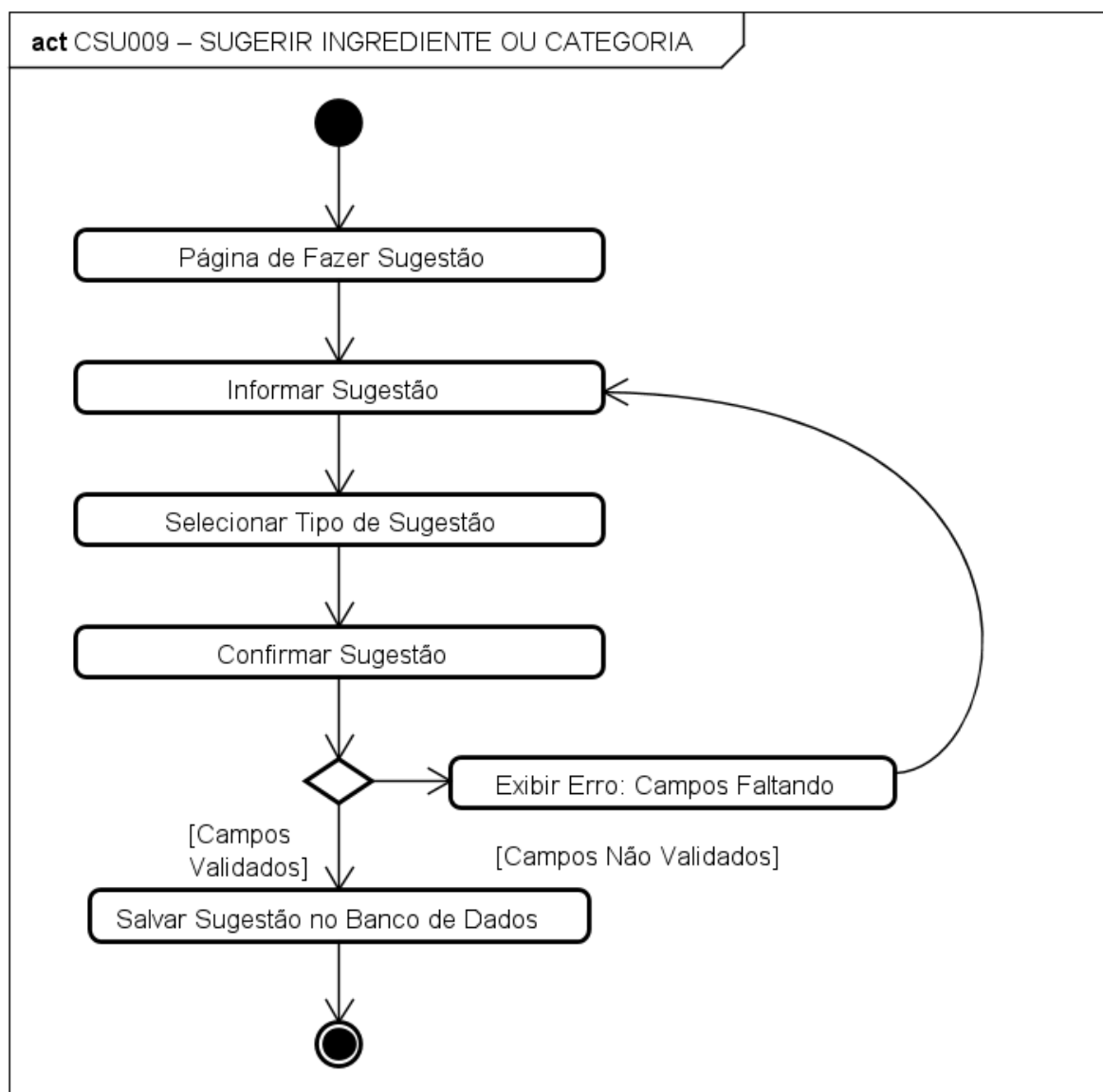
Figura 47 – Diagrama de Atividade – Sugerir Ingrediente ou Categoria
