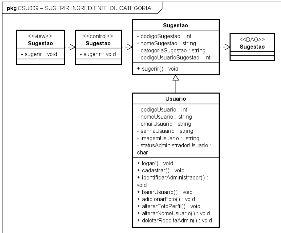
Figura 30 – Diagrama de Classes de Projeto – Sugerir Ingrediente ou Categoria
