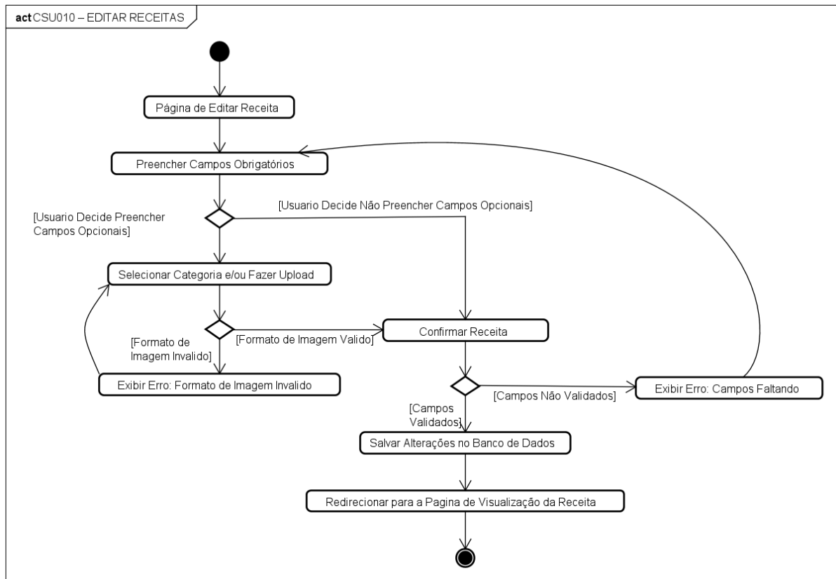
Figura 48 – Diagrama de Atividade – Editar Receitas
