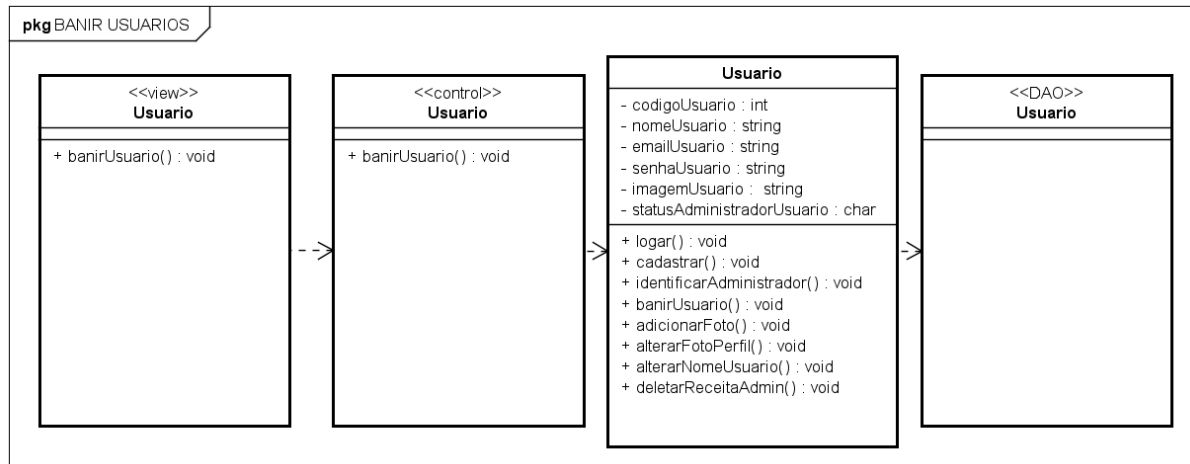
Figura 29 – Diagrama de Classes de Projeto – Banir Usuários
