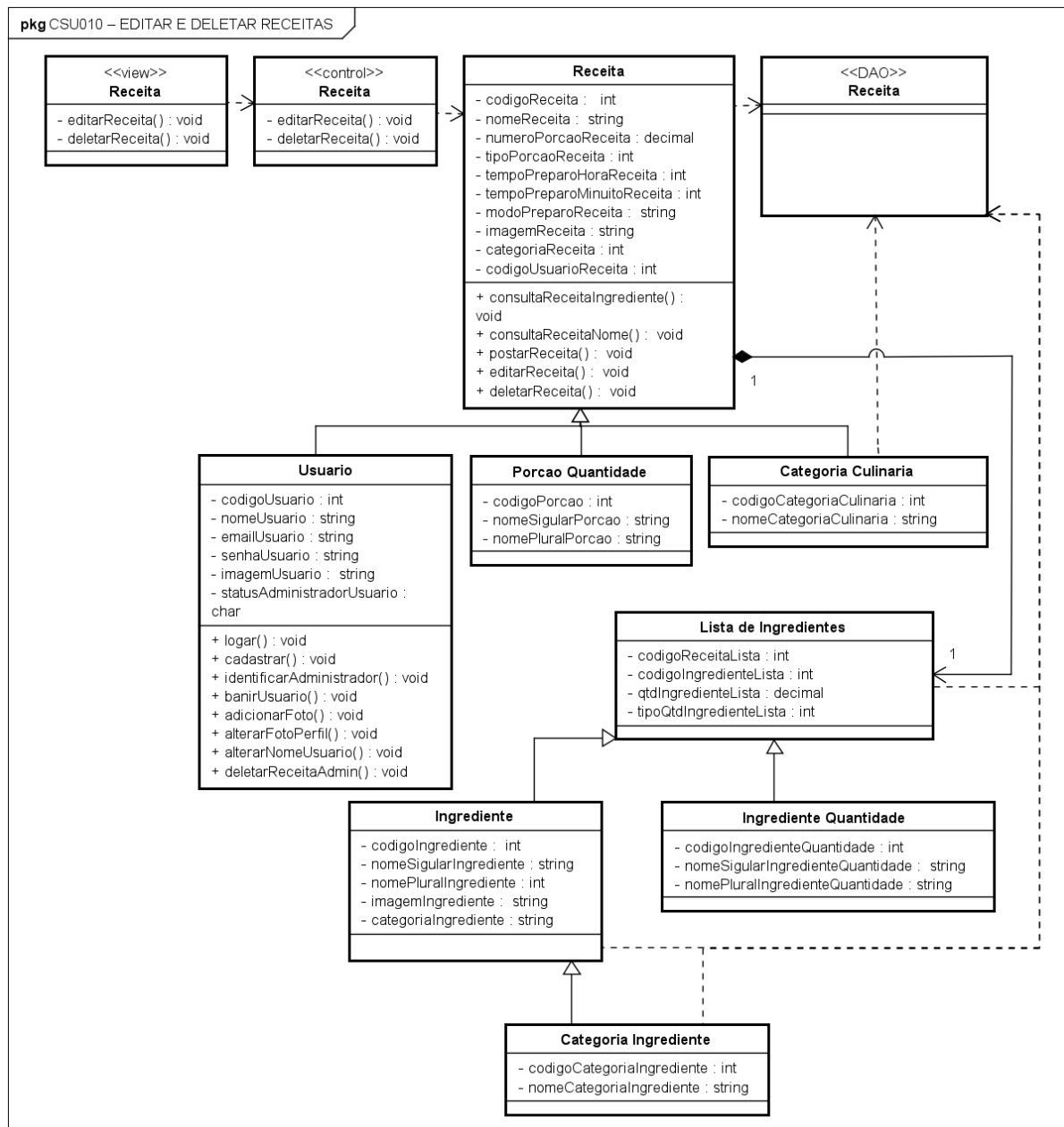
Figura 31 – Diagrama de Classes de Projeto – Editar e Deletar Receitas
