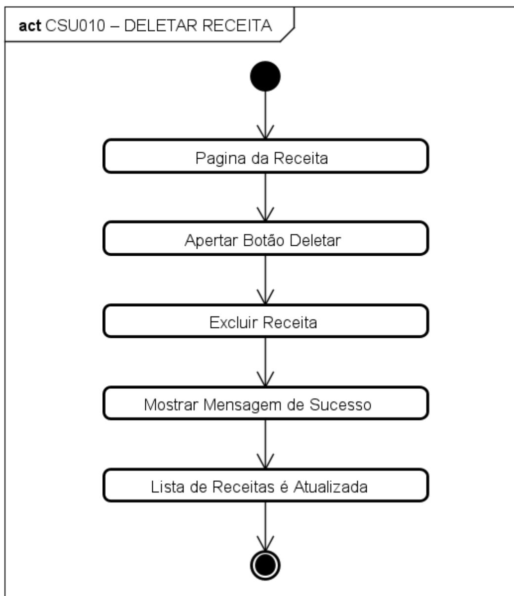
Figura 49 – Diagrama de Atividade – Deletar Receitas
