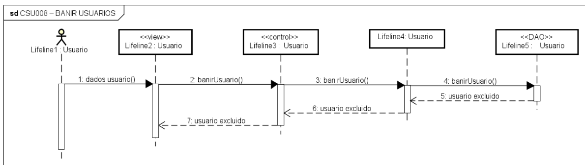
Figura 37 – Diagrama de Sequência – Banir Usuários
