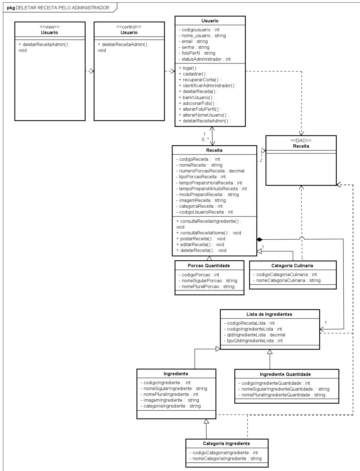
Figura 28 – Diagrama de Classes de Projeto – Deletar Receita Pelo Administrador
