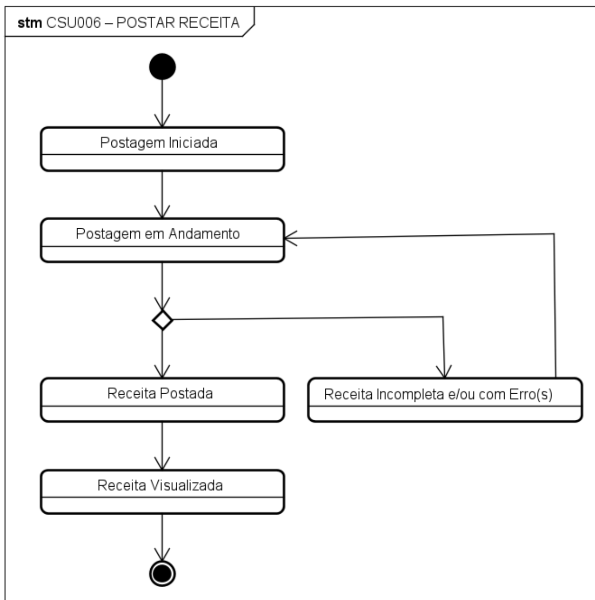
Figura 53 – Diagrama de Estado – Postar Receita
