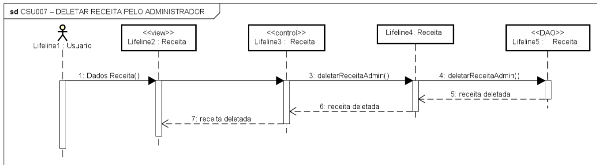
Figura 36 – Diagrama de Sequência – Deletar Receita Pelo Administrador
