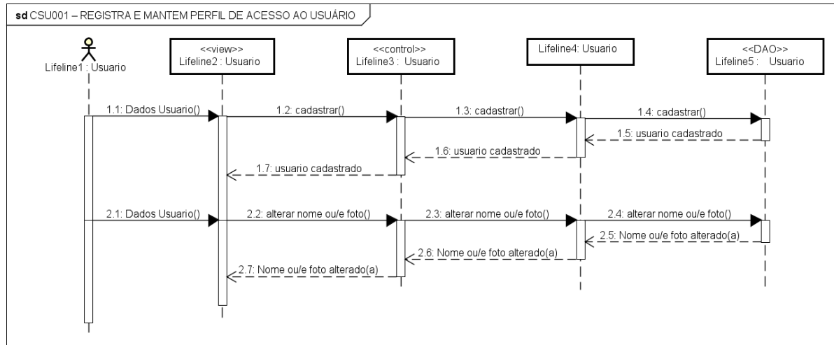
Figura 32 – Diagrama de Sequência – Registra e Mantem Perfil de Acesso ao Usuário.
