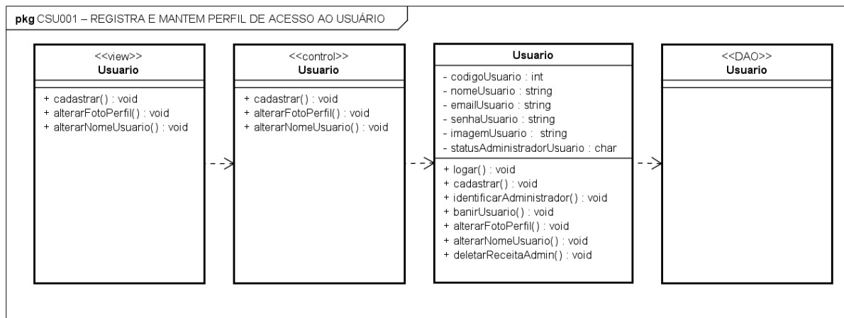
Figura 24 – Diagrama de Classes de projeto – Registra e Mantem Perfil de Acesso ao Usuário
