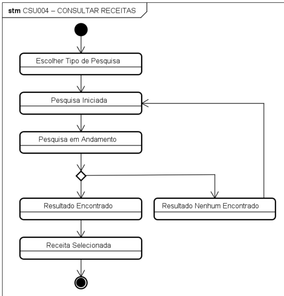
Figura 52 – Diagrama de Estado – Consultar Receitas
