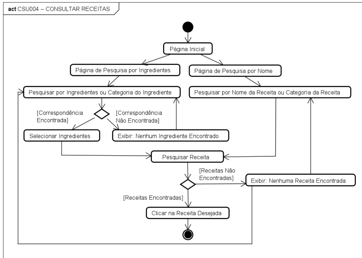
Figura 43 – Diagrama de Atividade – Consultar Receitas
