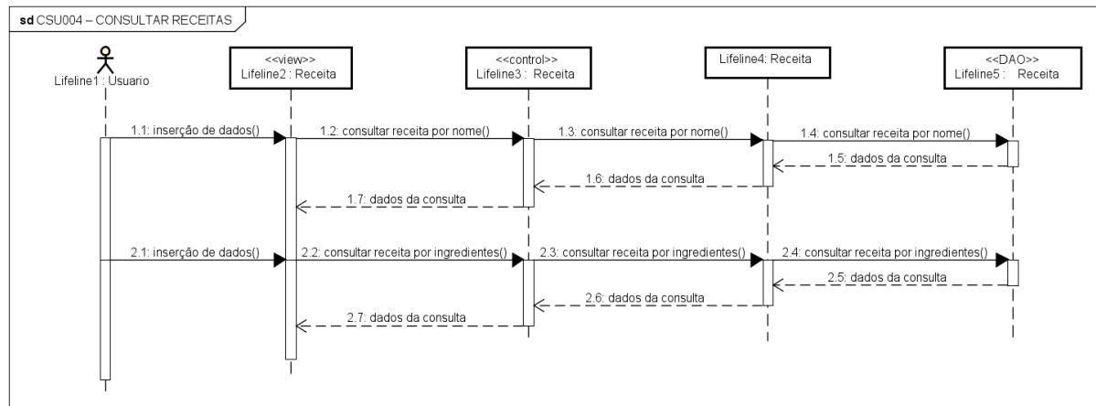
Figura 34 – Diagrama de Sequência – Consultar Receitas
