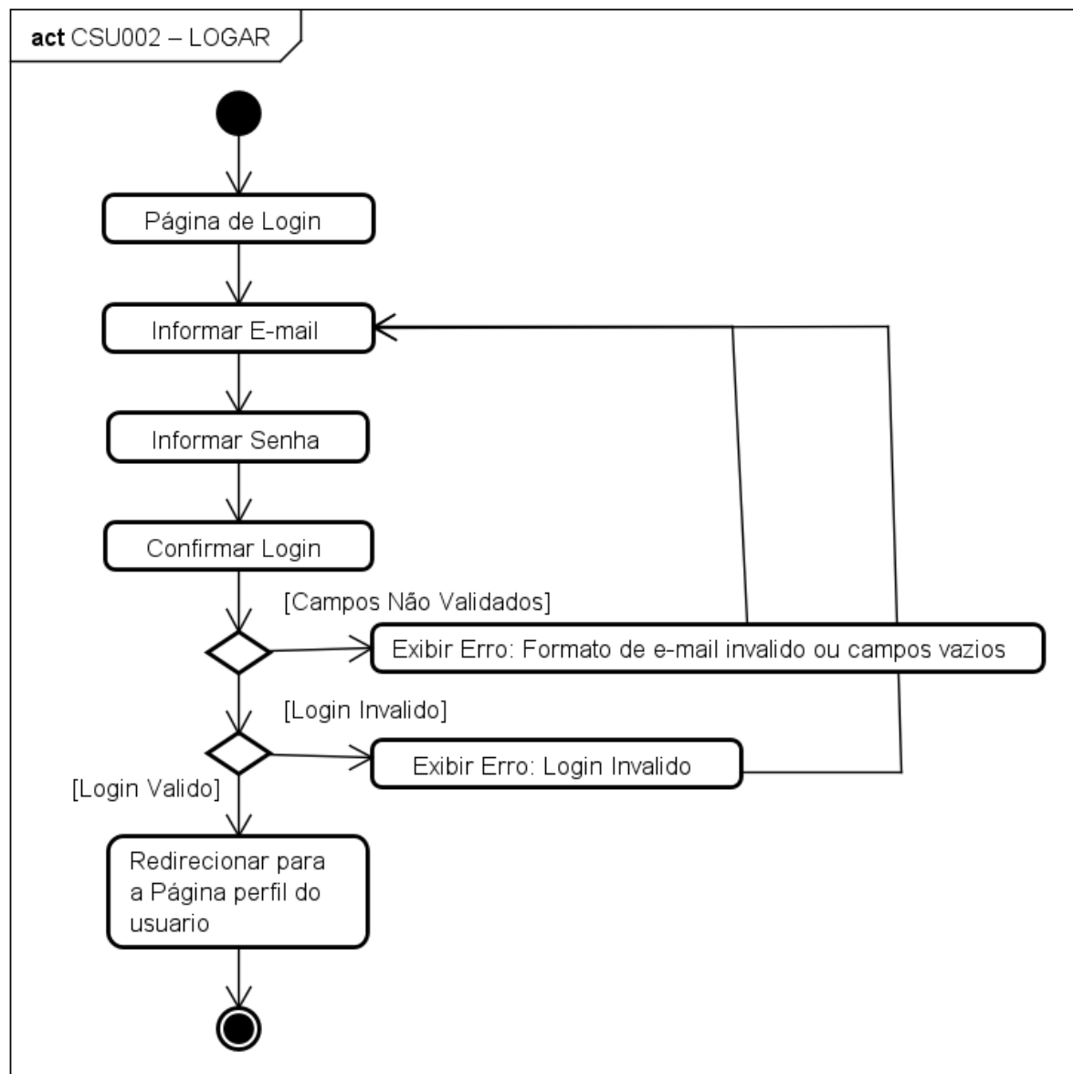
Figura 42 – Diagrama de Atividade – Logar
