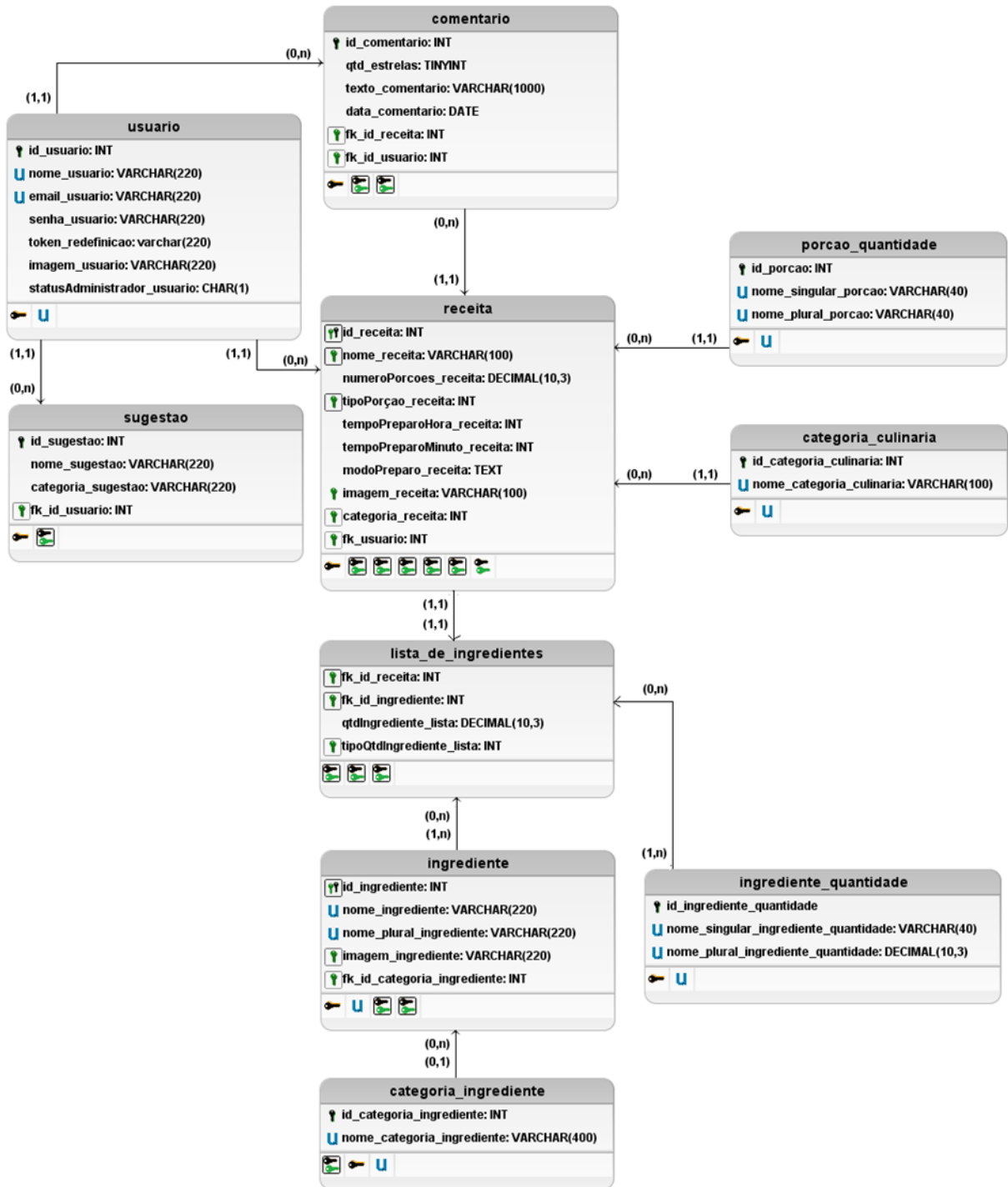
Figura 59 – Modelo Lógico de Base de Dados
