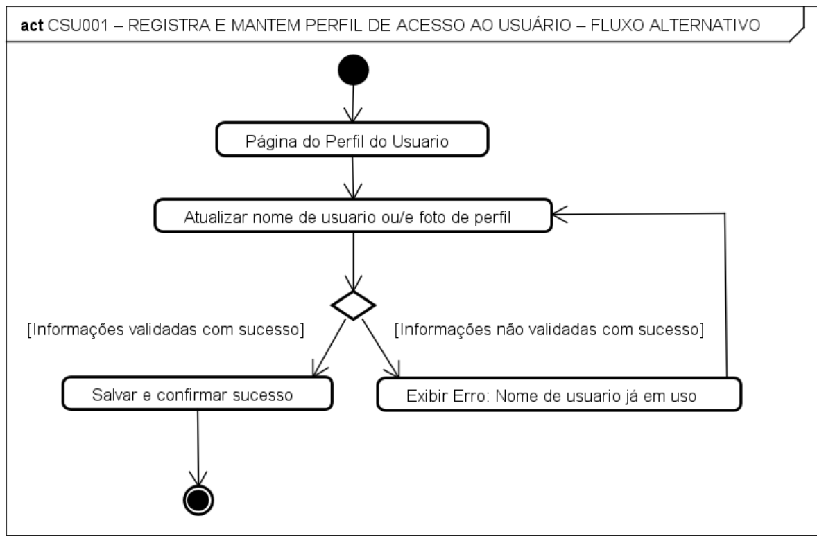
Figura 41 – Diagrama de Atividade – Fluxo Alternativo do Registra e Mantem Perfil de Acesso ao Usuário
